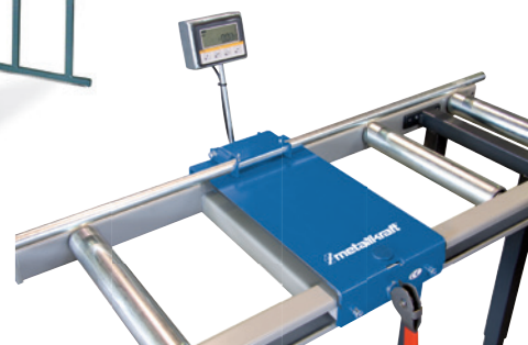
Fig. : MRB LC-E • Avec ruban magnétique de mesure, système d'affichage digital, chariot et butée montés sur roulement
