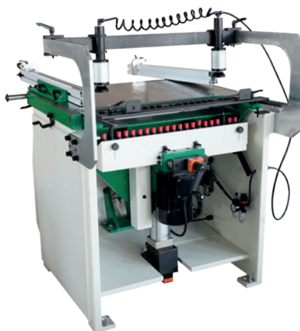
Fig. : MDB 21 • Vue arrière
