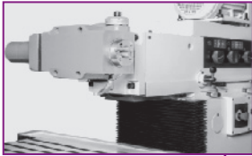
Tête de fraiseage · Pivotante à ± 90°
