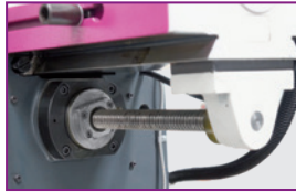
Dispositif de fraiseage horizontal · Pour les opérations de fraiseage en position horizontale
