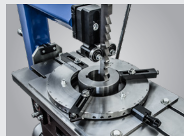
• Plateau diviseur gradué (accessoire optionnel n° d'art. : 388 9201) • Avec différentes graduations angulaires • Serrage et changement de serrage précis et rapide des pièces à usiner
